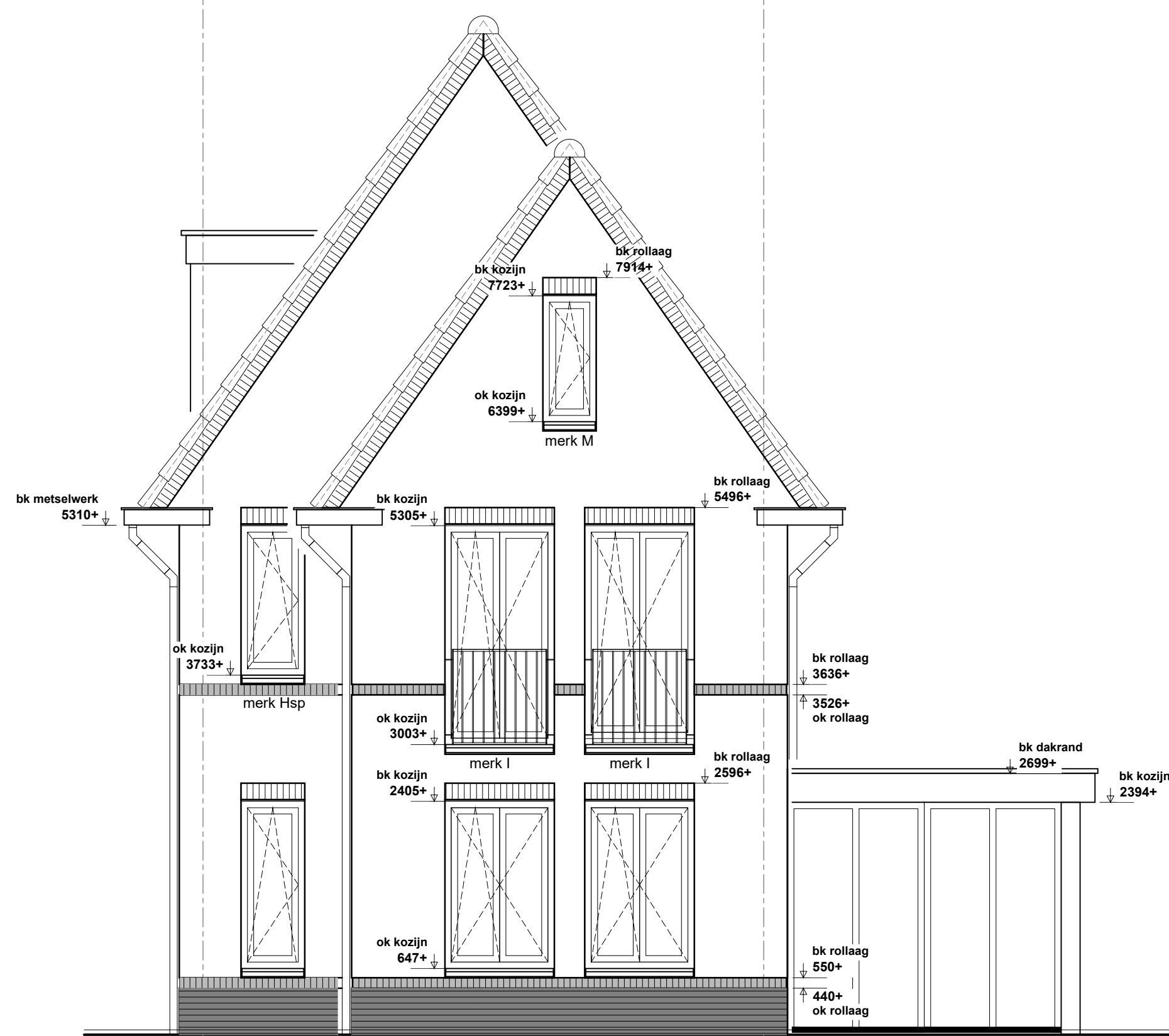
1 - voorgevel -
